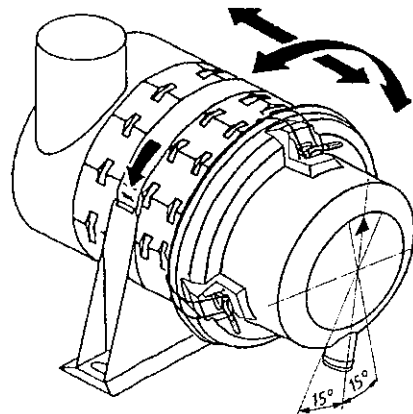
Ventil för dammtömning ska vara riktad nedåt
