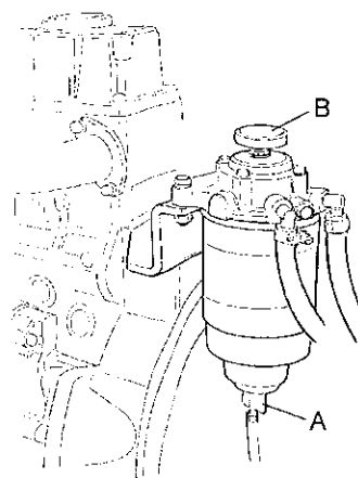
Bränslefilter med avluftningsventil
