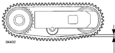
Band ska inte slacka mer än 10-15 mm
