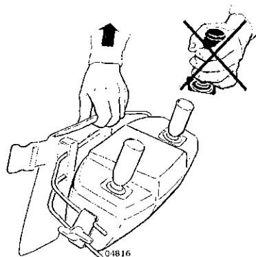
Bygel för lyft av manöverdon
