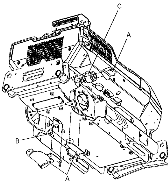
Tappa ur olja och byt oljefilter
