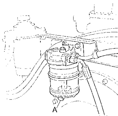
Dränera vattenavskiljaren med dränerskruv (A)
