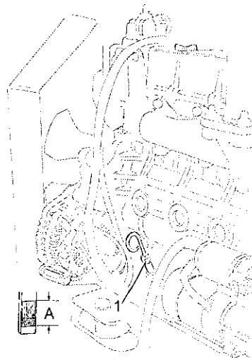
Kontroll av oljenivå
