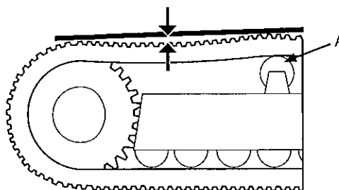
Bandsidor med överrulle (A)
