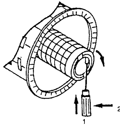
Bryt sekundärelementets försegling
