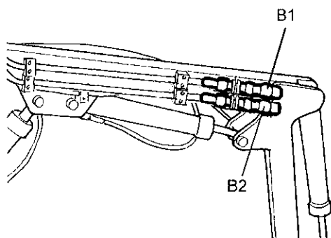
Anslutning av dubbelverkande redskap
