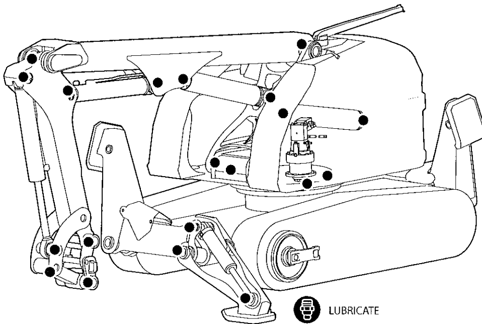
Symboler vid smörjramp B280
