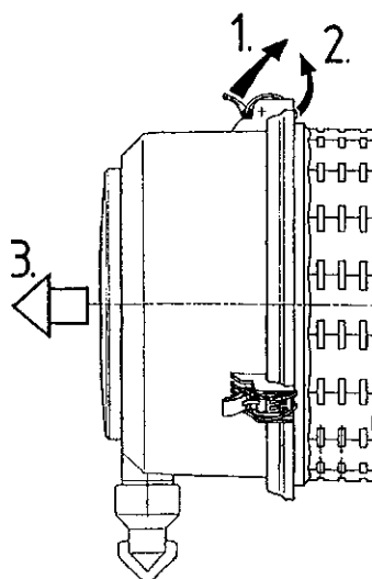
1 - 2 Lossa trådsträckarna, 3 Dra ut behållare
