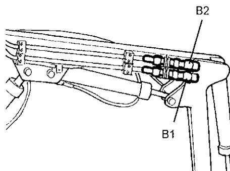
Anslutning av dubbelverkande redskap Brokk 260, Brokk 800
