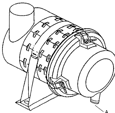
Öppna tappningsventil (A) för att avlägsna smuts- och damm
