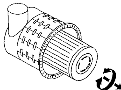
Vrid och dra ut filterelementet
