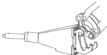
Bild 1. Utgångsläget vid redskapsbyte är att redskap med fästkrokar ska vara placerade enligt bilden.
