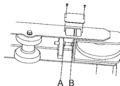
Bandspänning med justerskruv (B) och låsmutter (A)
